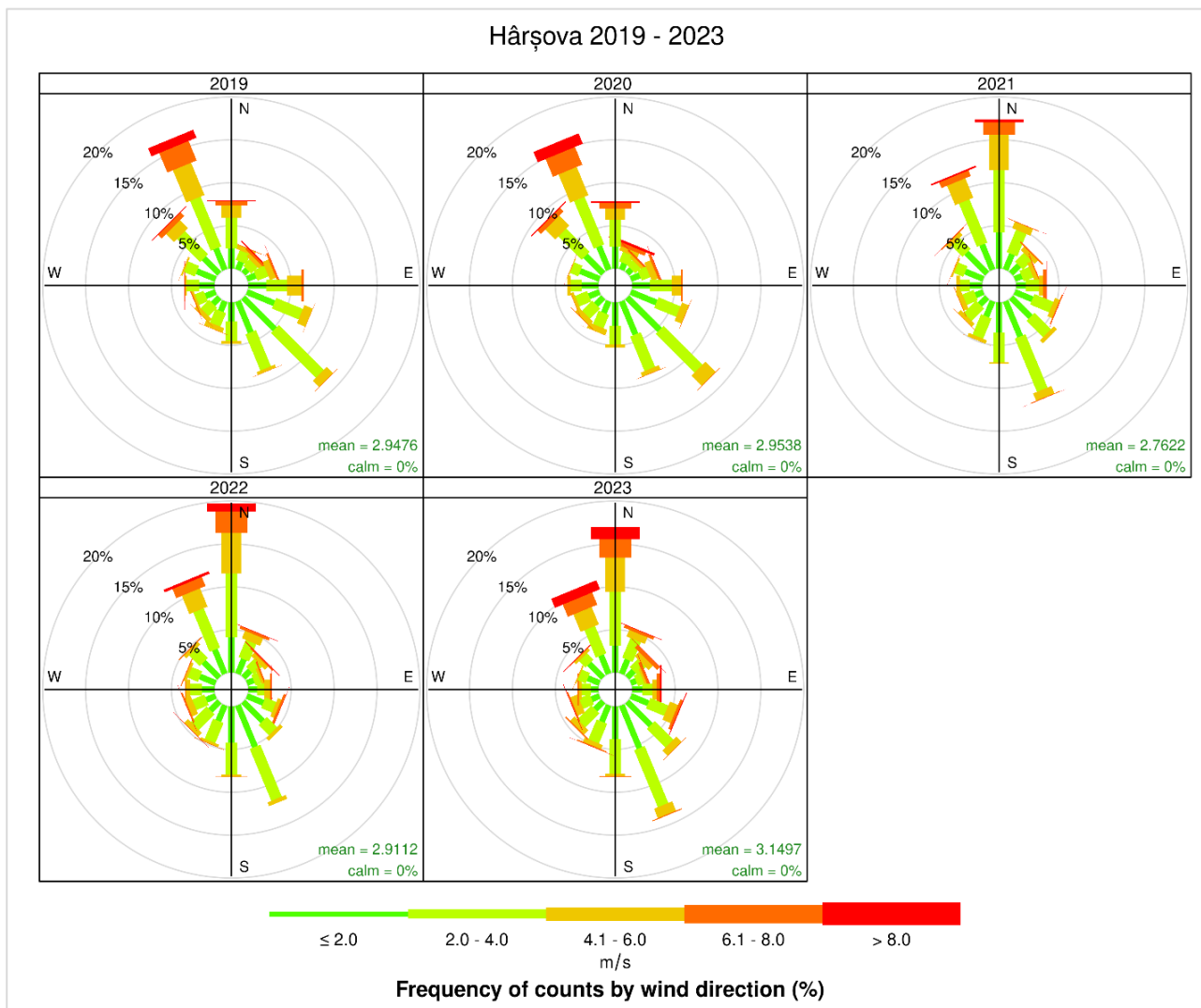
Figura 3-15: Frecvența medie anuală a vântului (%) la stația meteorologică Hârșova în perioada 2019 – 2023
